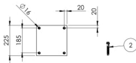
Rysunek techniczny:
